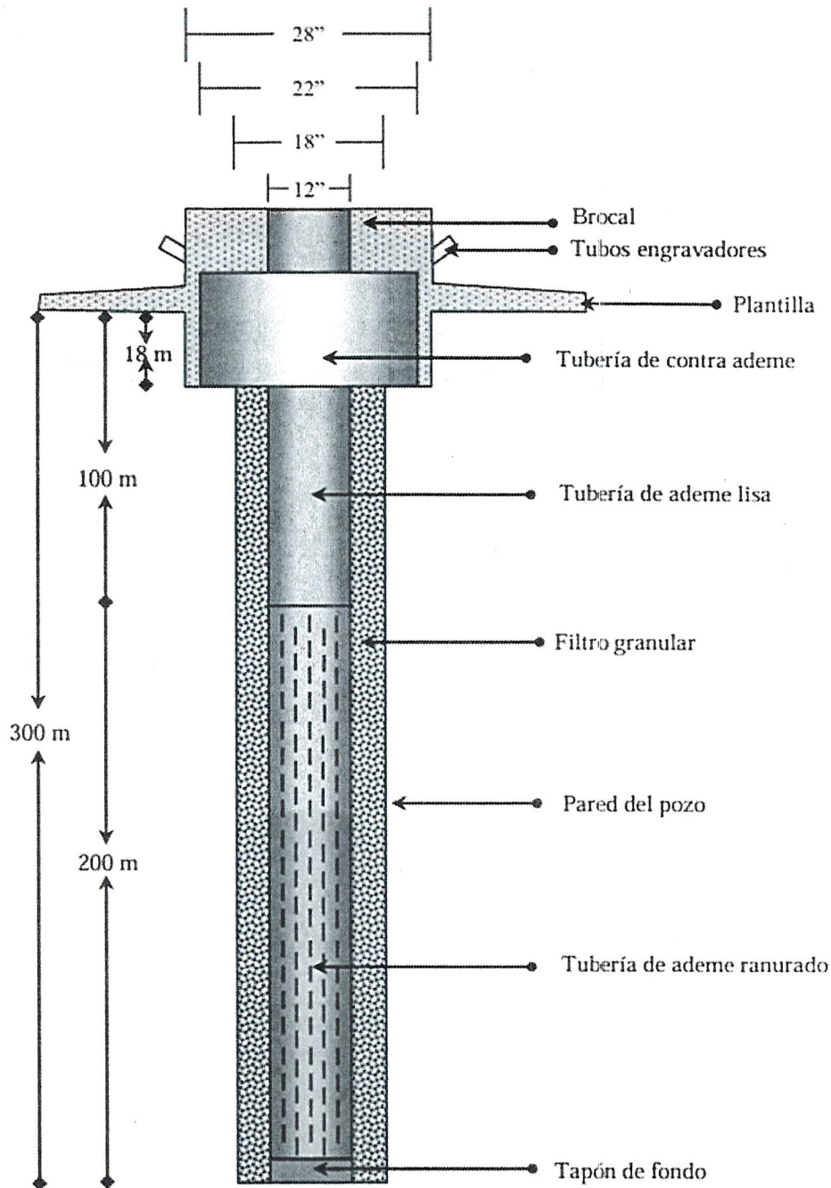
Ilustración 1.- Diseño constructivo del pozo para la Zona de Ojo Zarco
