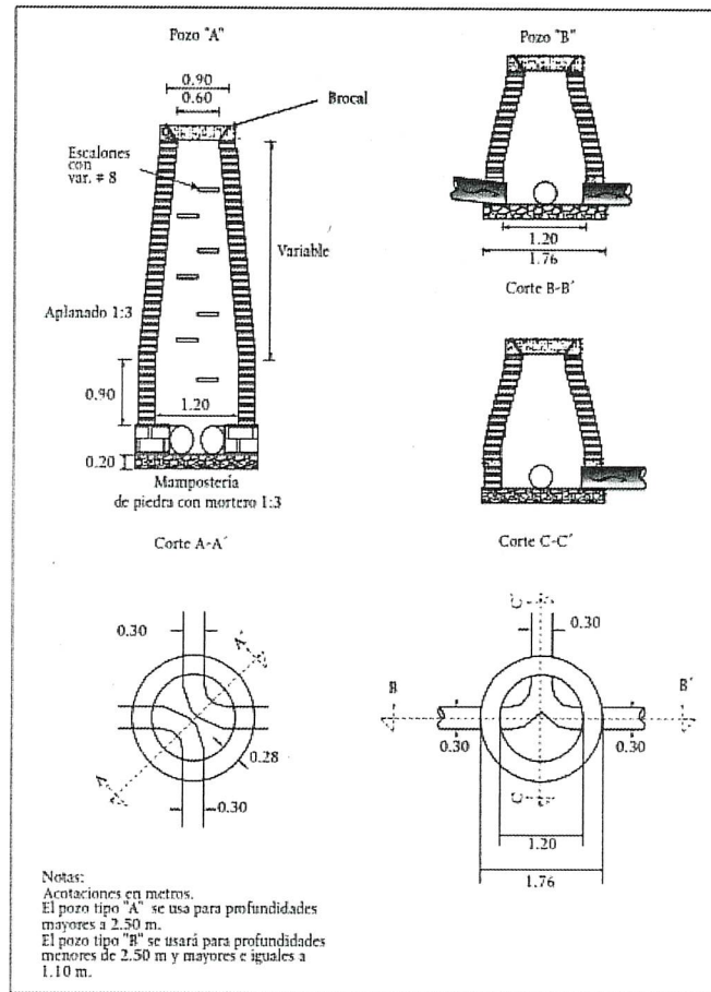
Fig. 1.- Pozos de visita común. Fuente: M.A.P.A.S. libro 19.
