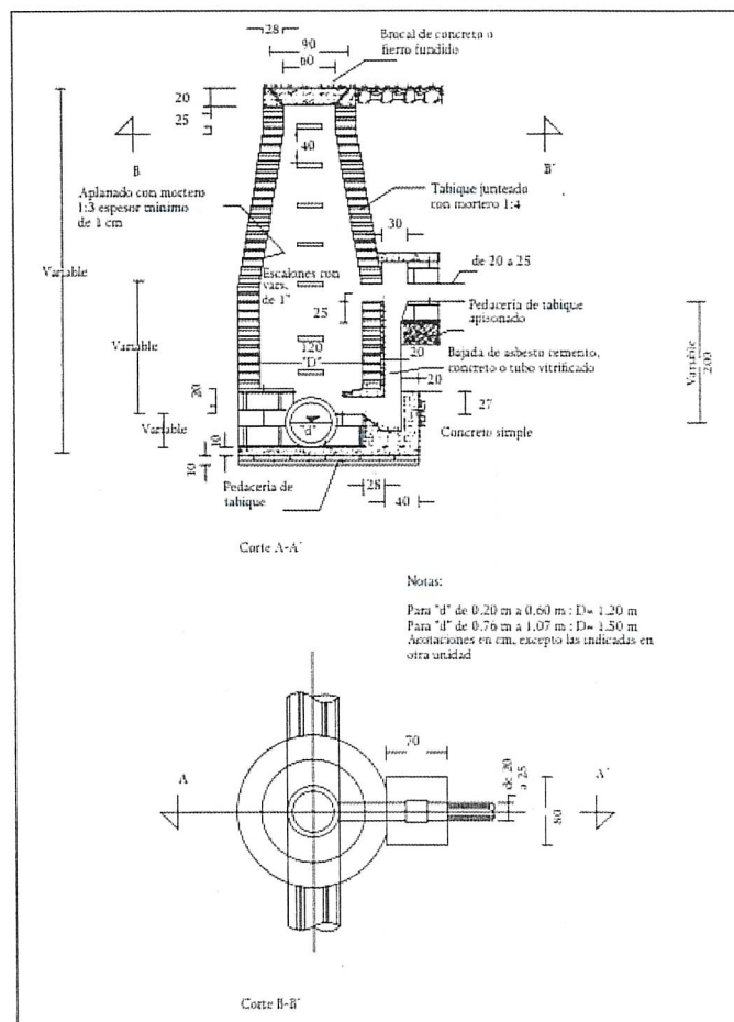
Fig. 2.- Pozo con caída adosada. Fuente: M.A.P.A.S. libro 19.
