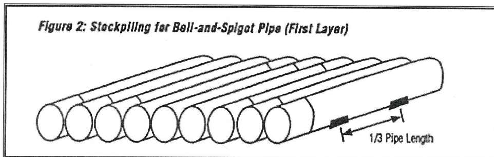
Fig. 2.- Detalle de almacenamiento de la tubería.
