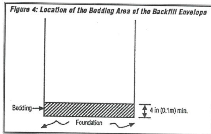
Fig. 4.- Encamado de la tubería.
