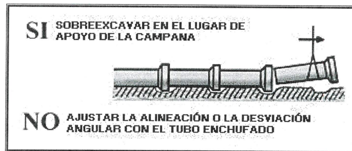
Fig. 6.- Detalle de la campana en tuberías.
