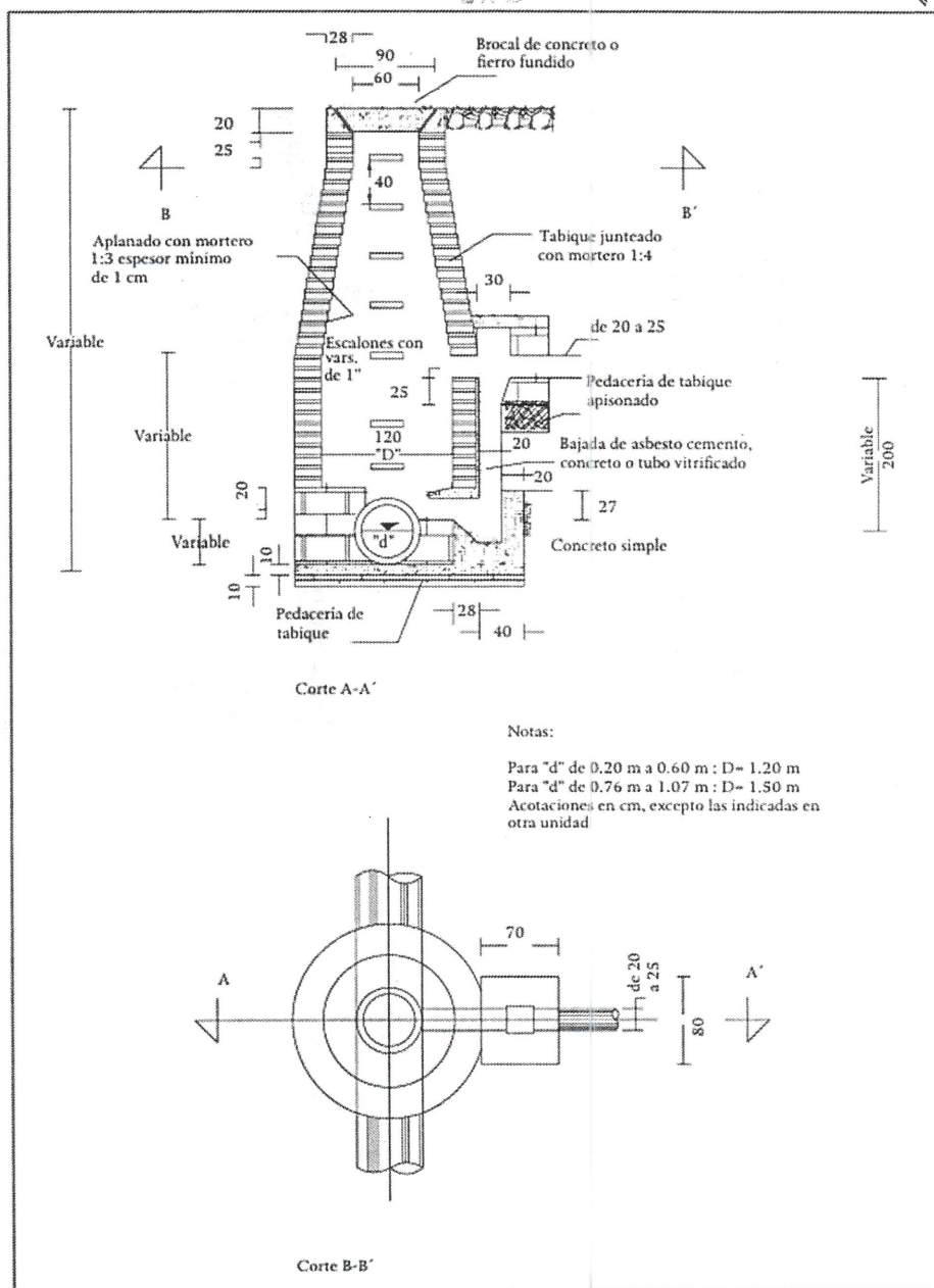
Fig. 2.- Pozo con caída adosada. Fuente: M.A.P.A.S. libro 19.
